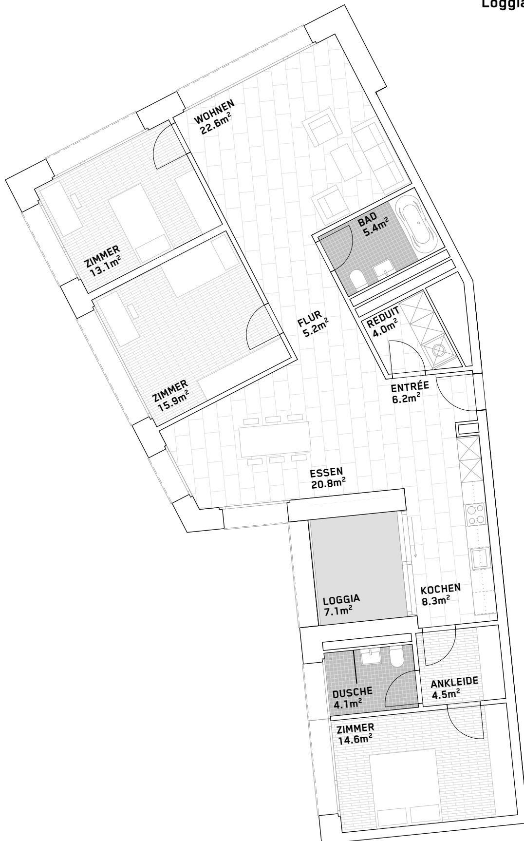
Grundriss 1:100
